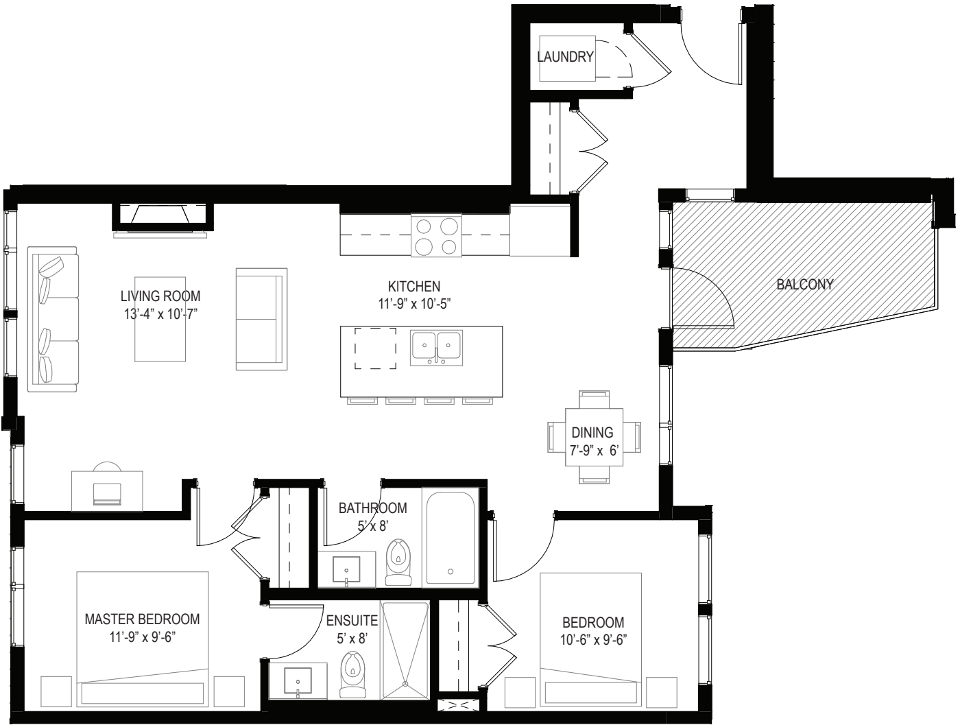
2 BDRM - TYPE G 988 SF
